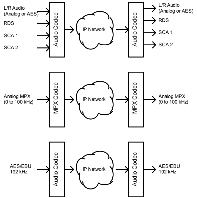
FIG 5 STL TOPOLOGIES
